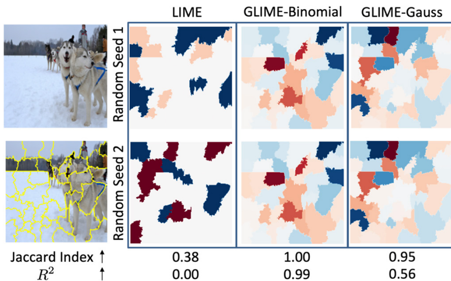
图 1: 在使用两个随机种子的小型 Swin-Transformer 上，对 ImageNet 图像进行 LIME 和 GLIME 解释。使用 \sigma=0.25 和样本大小为 16384。第二行下方呈现的数值代表两个解释图之间的 Jaccard 指数。
