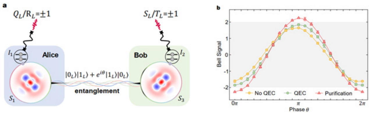
图 3 利用纠缠的逻辑量子比特演示贝尔不等式的违背
